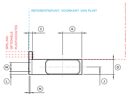
ZIJAAANZICHT
