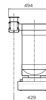
VOORAANZICHT
