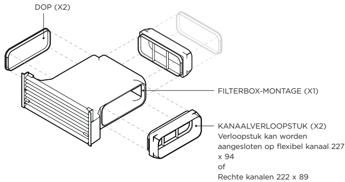
GEDETAILLEERD ISOMETRISCH AANZICHT
