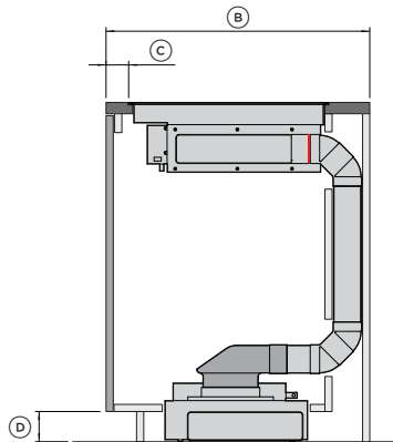
ZIJAANZICHT
