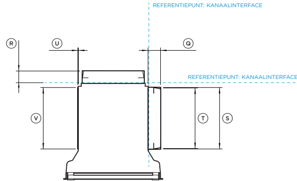
BOVENAANZICHT
