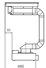
ZIJAANZICHT
