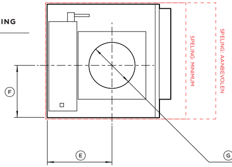
ONTWERPWEERGAVE
