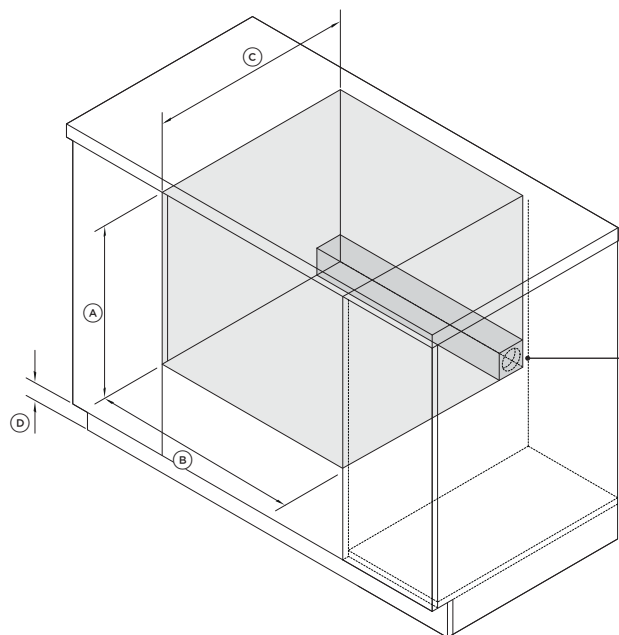
ISOMÉTRIQUE
