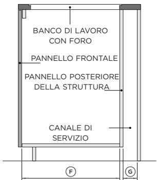
VISTA LATERALE
