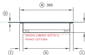
VISTA FRONTALE
