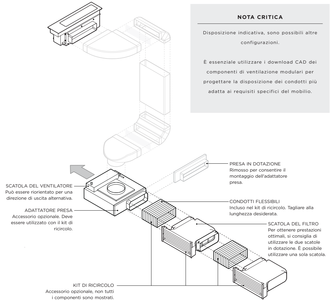
PANORAMICA CON COMPONENTI DEI CONDOTTI CON RICIRCOLO
