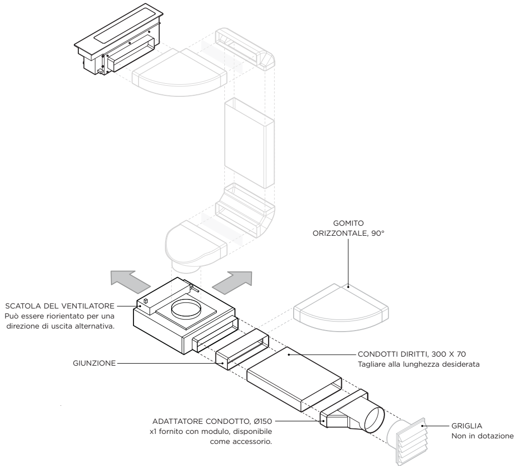
PANORAMICA CON COMPONENTI DEI CONDOTTI
