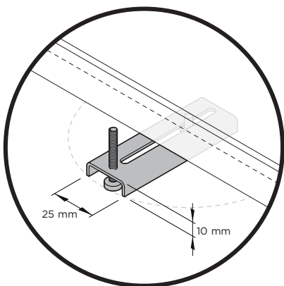
DETTAGLIO A
