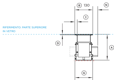
VISTA FRONTALE
