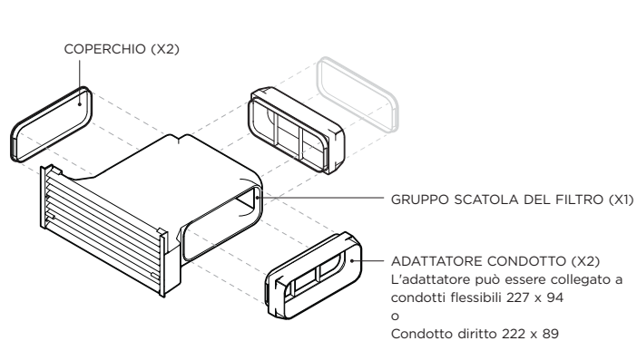
VISTA ISOMETRICA ESPLOSA
