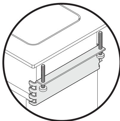
DETTAGLIO B
