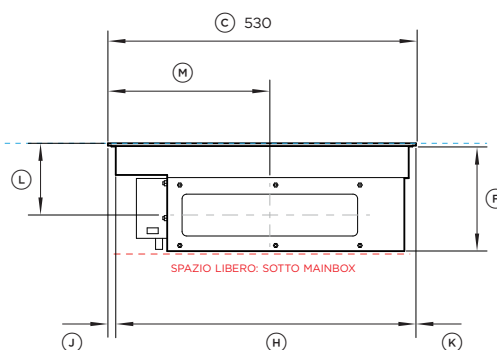
VISTA PROFILO
