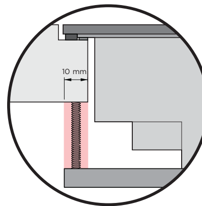
DETTAGLIO C
