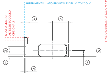
VISTA PROFILO
