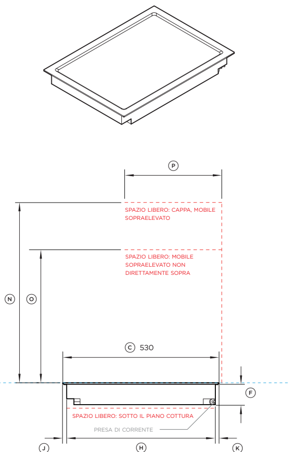
VISTA PROFILO
